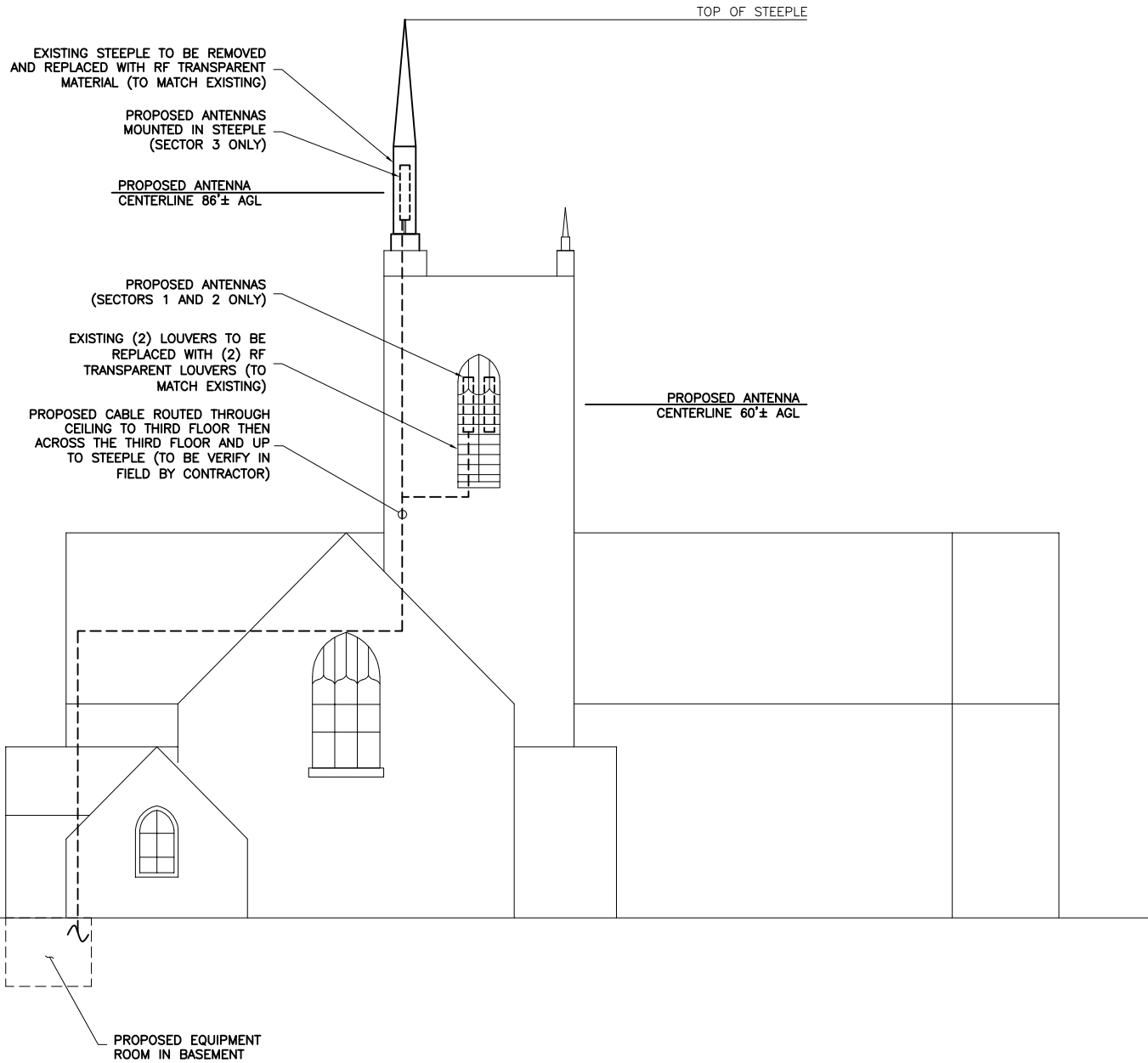
1 LE-3 ELEVATION SCALE: 1" = 20'
